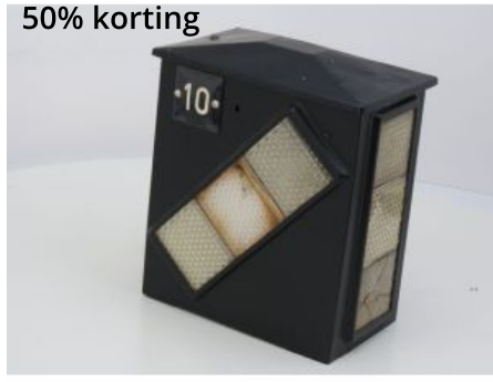
Wissel Lantaarn No 10
